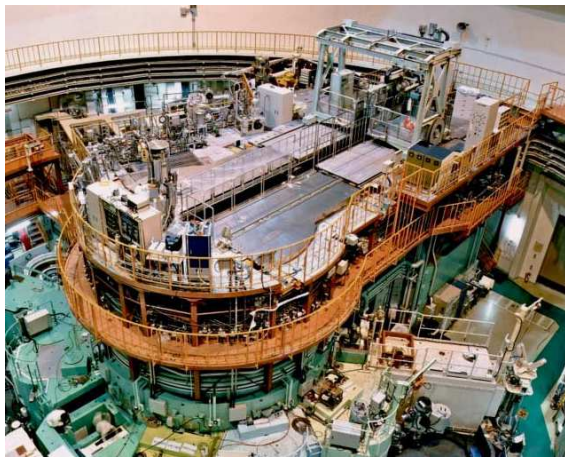
原子炉 (JRR-3)
